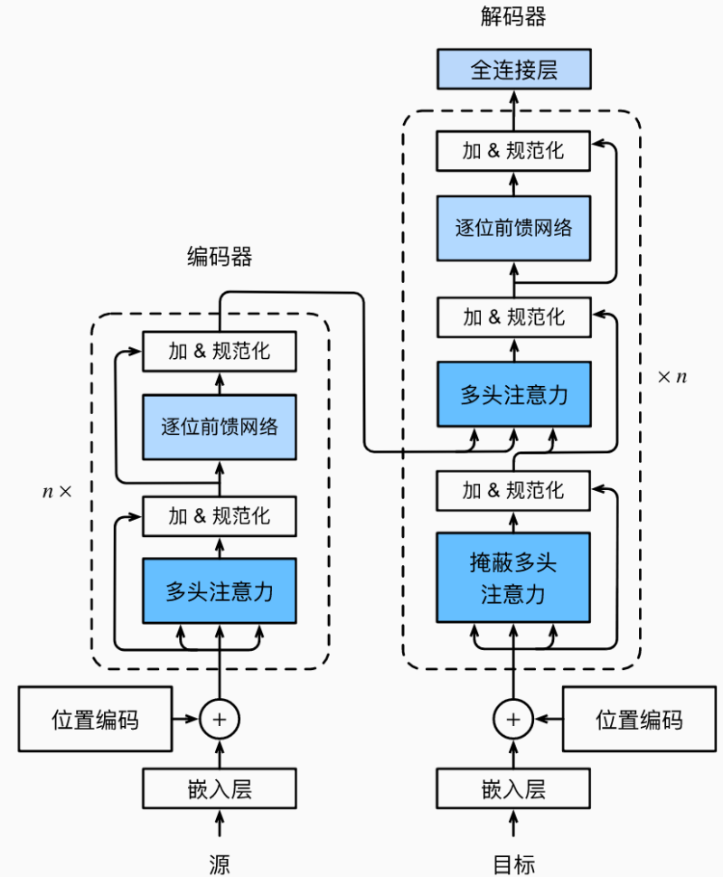
图10.7.1 transformer架构
