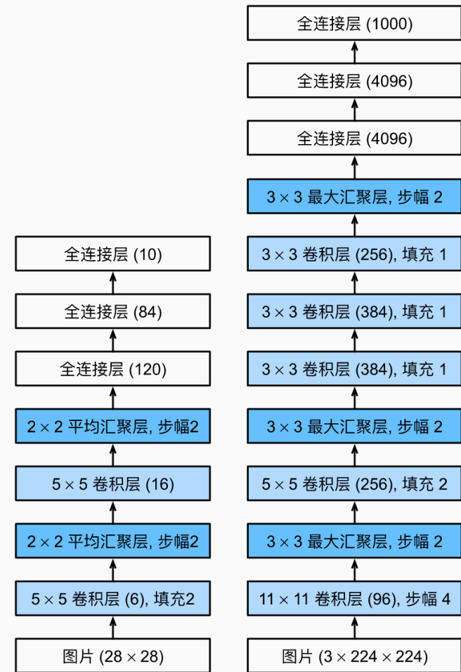
图7.1.2 从LeNet (左) 到AlexNet (右)
