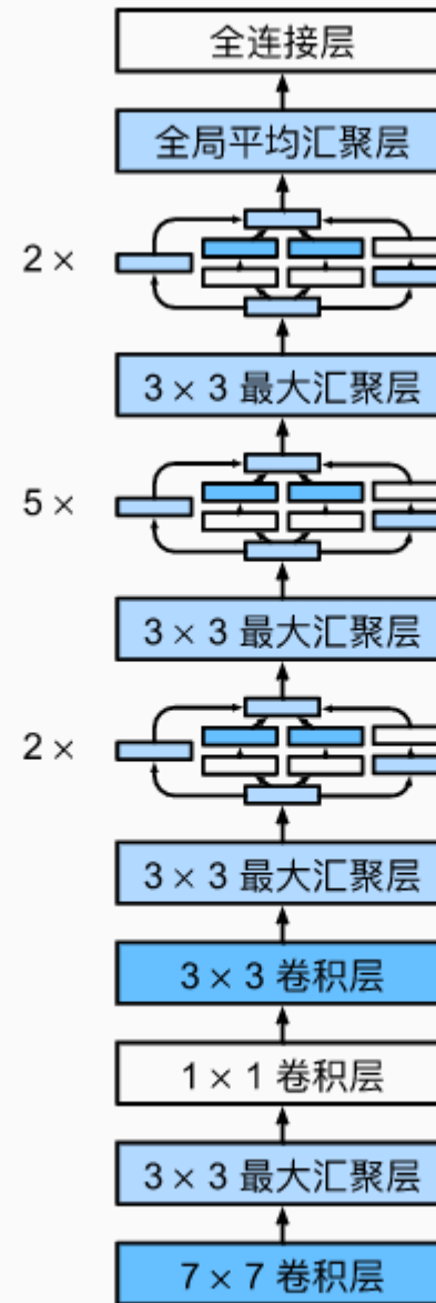
图7.4.2 GoogLeNet架构。
